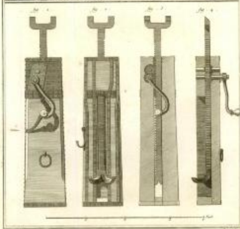
Sculpture L'opération de briser un bloc de Marbre et de Carre.
