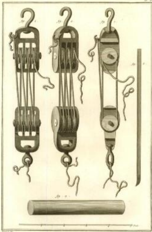
Sculpture, Mouffles, Ponce et Rouléau pour élever le Marbre
