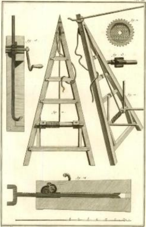
Sculpture, Instrumens qui servent à monter le marbre.
